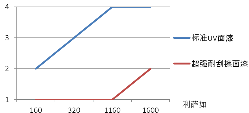
MSR-B (DIN EN 16094 – 马丁代尔测试)
